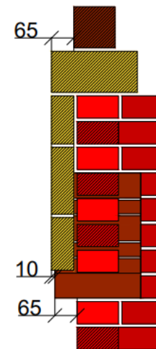
Разрез 1-1
